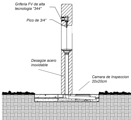
Vista Lateral
