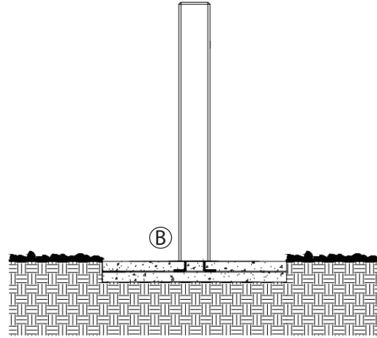
Vista Lateral
