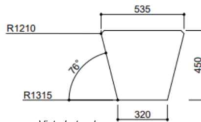
Vista Lateral
